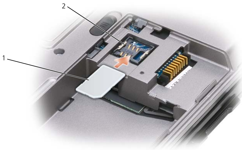
1 SIM カード 2 金属製ブラケット (2)
