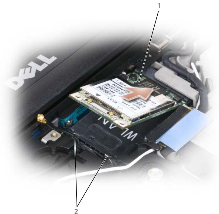
1 ワイヤレス LAN カード 2 金属製固定タブ (2)
